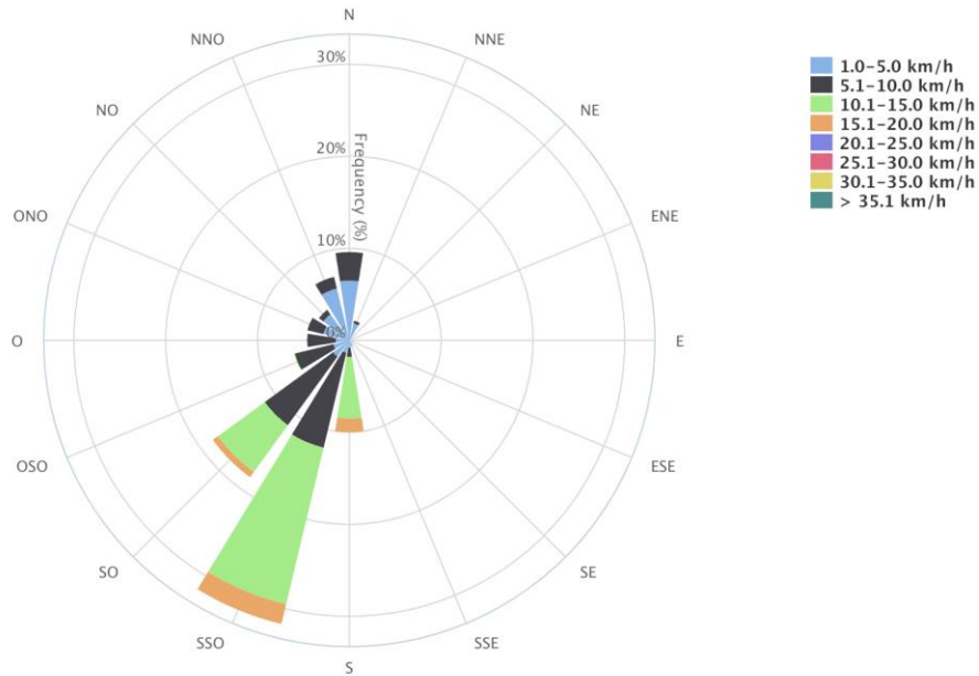
Figura 19. Distribución de la velocidad en la estación S02.
