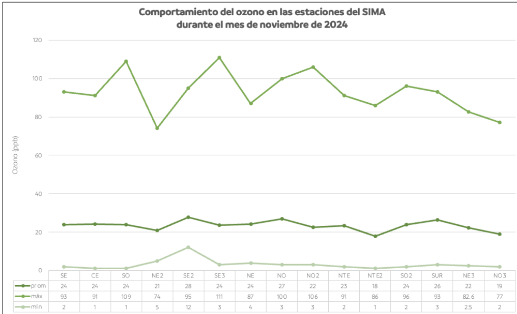
Figura 24. Comportamiento mensual del ozono en la ZMM.
