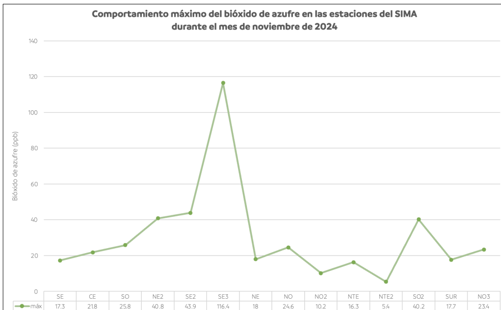
Figura 25. Comportamiento mensual de los máximos del bióxido de azufre en la ZMM.
