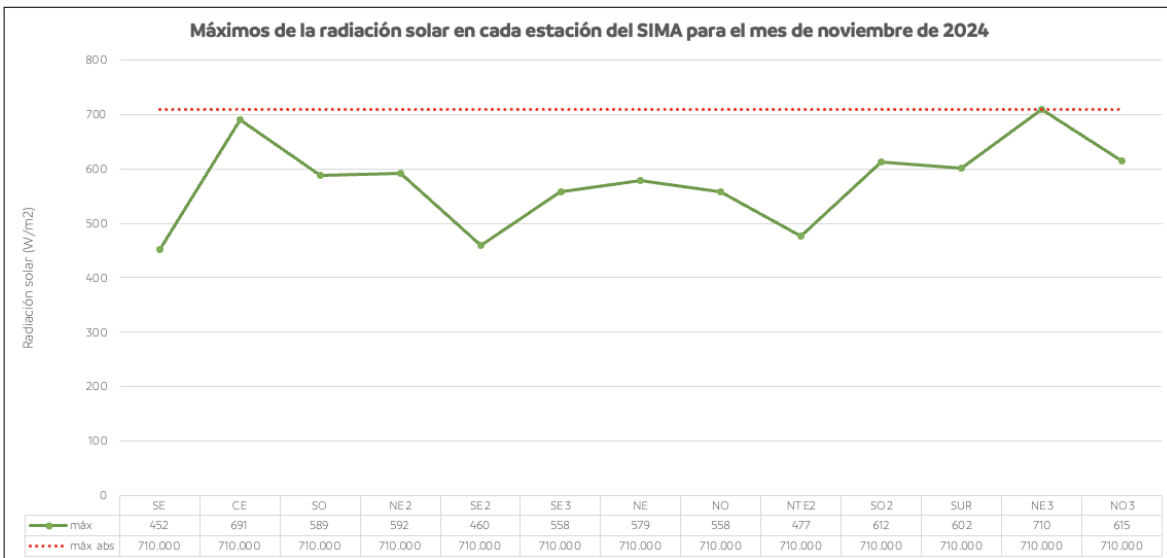
Figura 6. Comportamiento mensual de la radiación solar sobre la ZMM.
