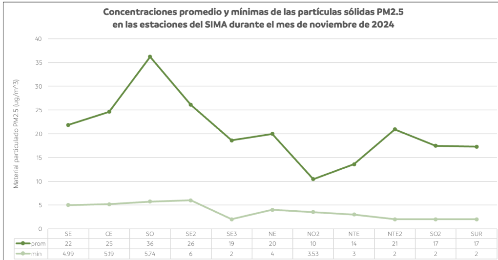
Figura 32. Comportamiento mensual promedio y mínimo de PM 2.5 en la ZMM.
