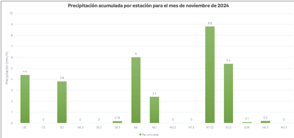
Figura 7. Acumulación de precipitación en estaciones del SIMA.
