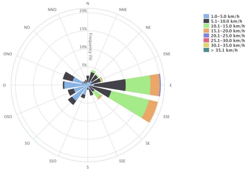
Figura 9. Distribución de la velocidad en la estación SE.
