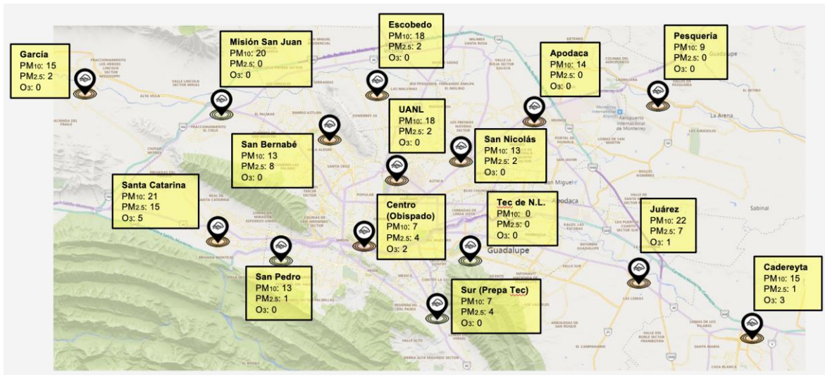
Figura 34. Días superiores al límite normado por estación del SIMA.
