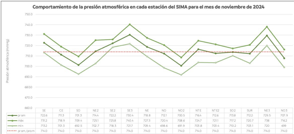
Figura 5. Comportamiento mensual de la presión atmosférica en la ZMM.
